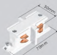
4 wire square I mini Connector EAN : 69012120 LU-TR4XMI-B White
